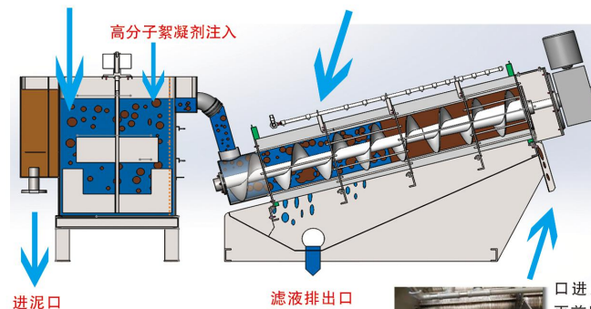
通过计量后的污泥在絮凝混合槽内与注入的高分子絮凝剂充分混合搅拌,形成良好的矾花。
